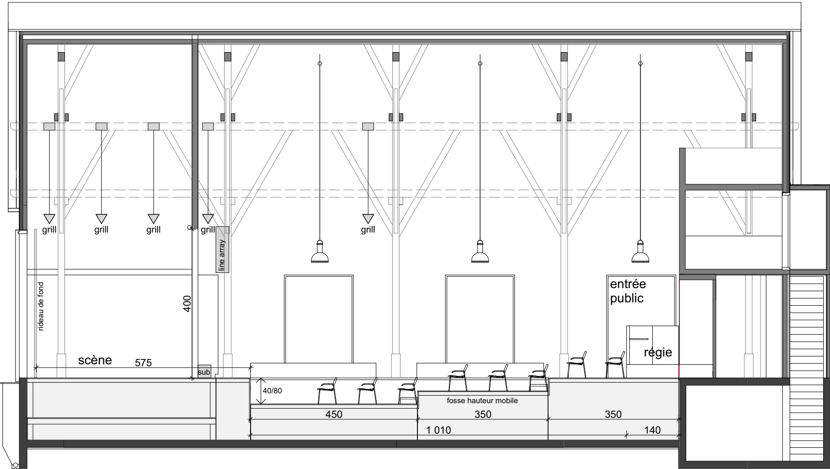
coupe longitudinale
